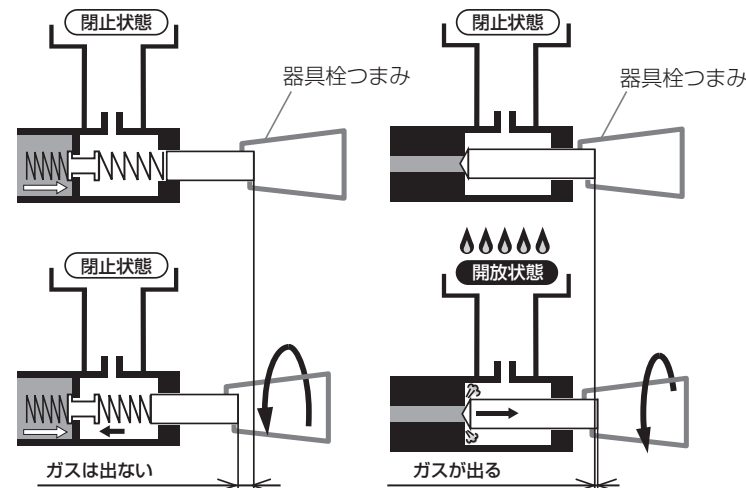
マイクロレギュレーターストーブ ウインドマスター SOD-310
